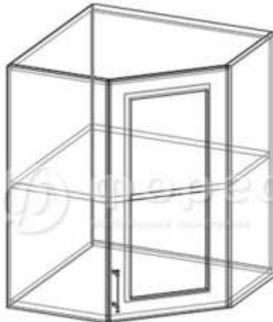
ШВУС-590 (ШxBxГ) 590x716x590 мм
