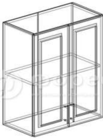
ШВС-600 (ШxBxГ) 600x716x314 мм
