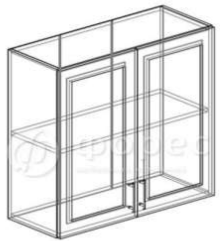
ШВС-800 (ШxBxГ) 800x716x314 мм
