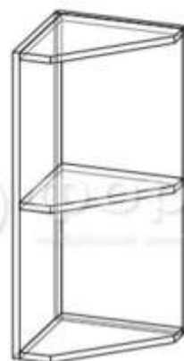
ШВПУ-300 (ШxBxГ) 284x716x298 мм
