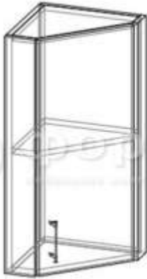
ШВТ-300 (ШxBxГ) 300x716x314 мм
