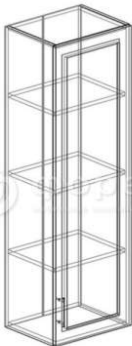
ШВПС-400 (ШxBxГ) 400x1292x314 мм
