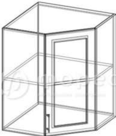
ШВУС-557 (ШxBxГ) 557x716x557 мм
